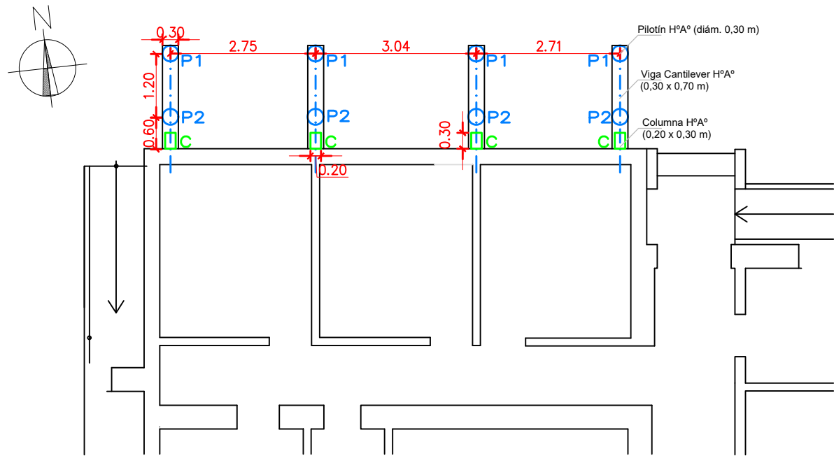
PLANTA REFUERZO ESTRUCTURAL - NIVEL +0.00 ESC 1:100
