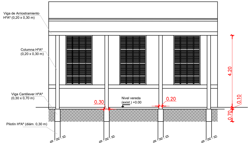
FACHADA NORTE - INTERVENCIÓN ESC 1:100
