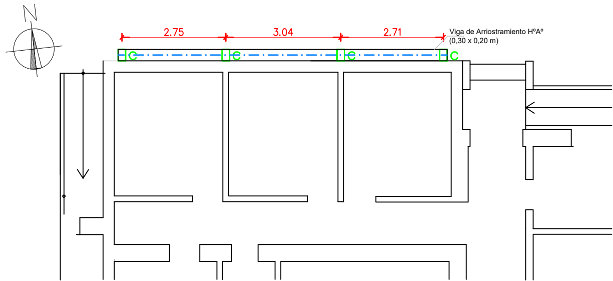
PLANTA REFUERZO ESTRUCTURAL - NIVEL +4.20 ESC 1:100
