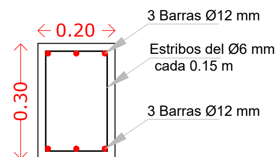
DETALLES CONSTRUCTIVOS ESC 1:10
