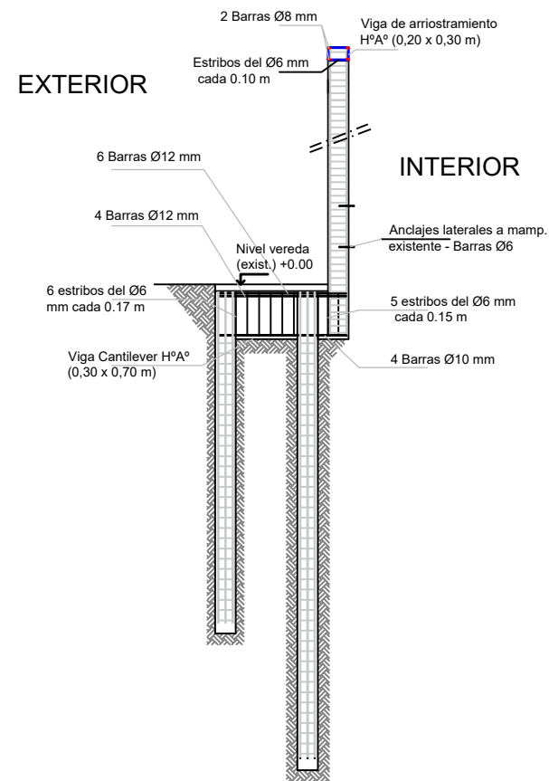
DETALLES CONSTRUCTIVOS ESC 1:100
