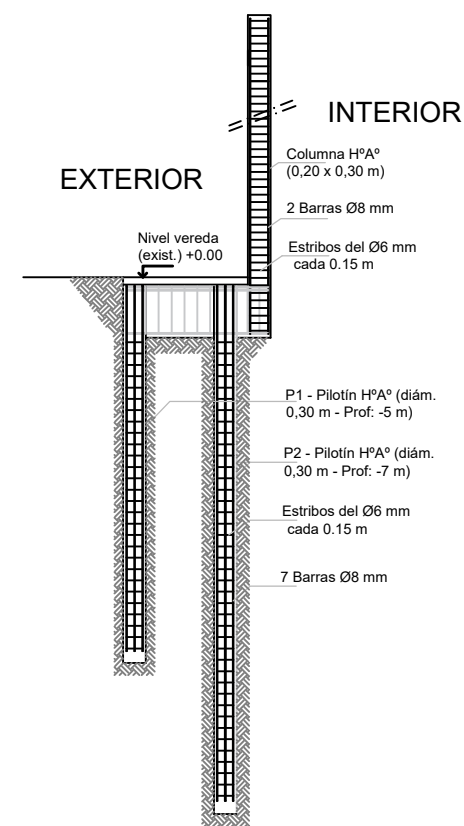
DETALLES CONSTRUCTIVOS ESC 1:100
