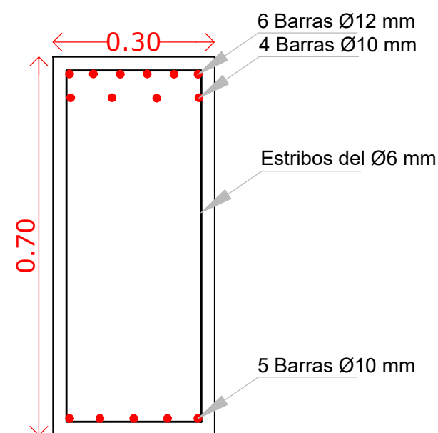
Detalle Viga Cantilever
