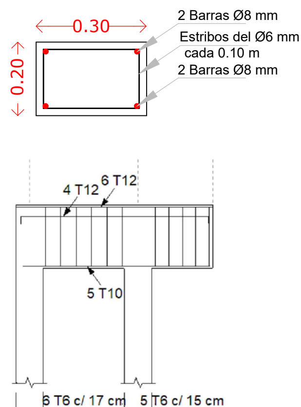
Detalle Vigas de Arriostamiento
